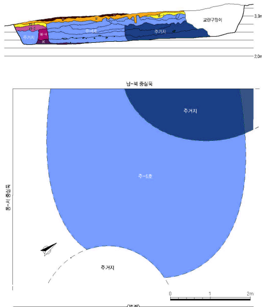
그림 5. 6호주거지 평면도 및 토층도 (국립문화재연구소 2013 p46)
